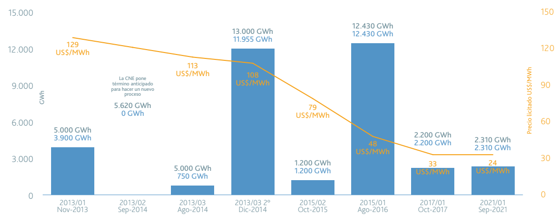
Figura 2.3: Resultados de licitaciones realizadas desde 2013 en adelante
