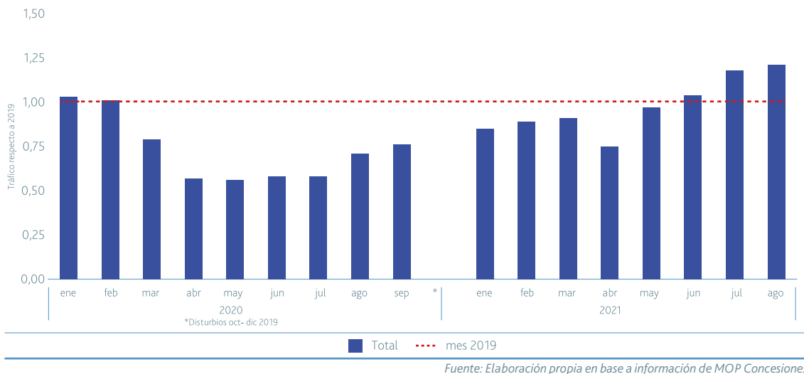
Figura 4.2: Tráfico interurbano durante pandemia versus 2019
