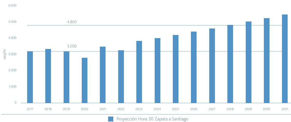
Figura 4.7: Proyección Hora 30 plaza de peaje Zapata sentido a Santiago (R68)
