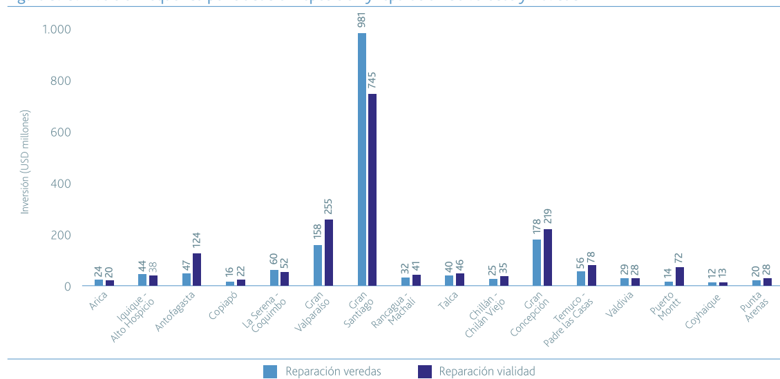
Figura 5.15: Inversión requerida por ciudad en reposición y reparación de veredas y vialidad
