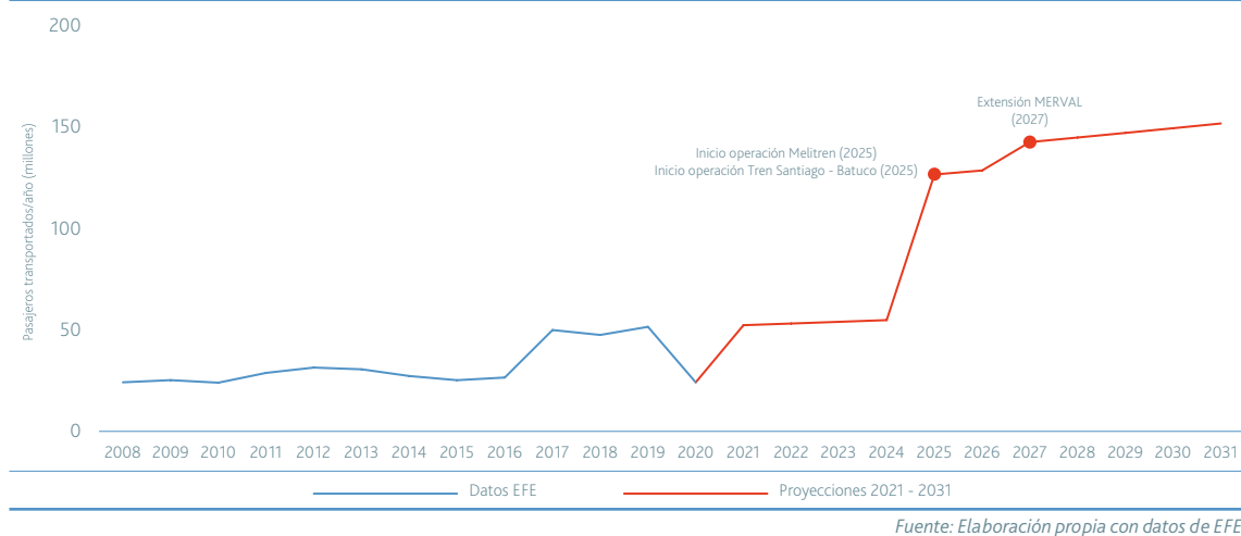
Figura 8.6: Proyección de demanda de pasajeros, período 2021 – 2031
